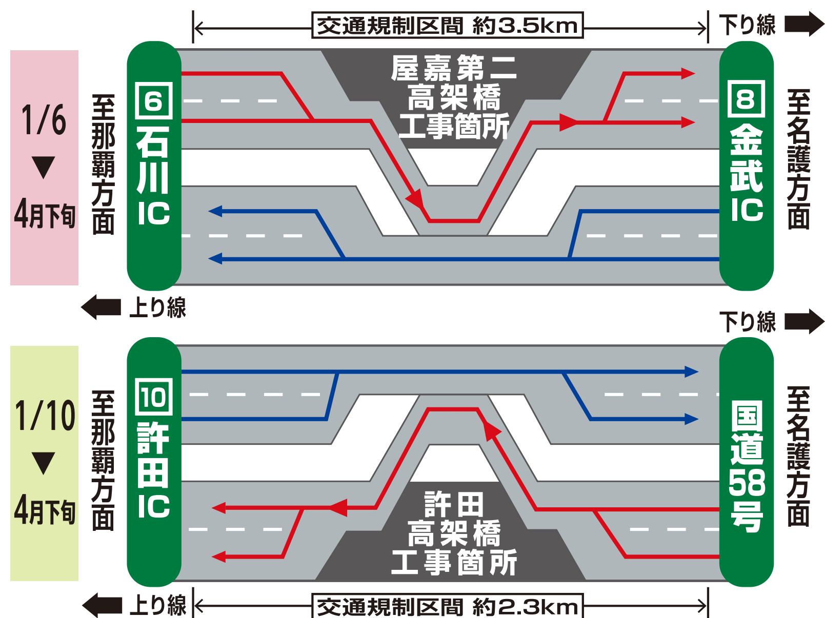
橋梁(床版取替)
