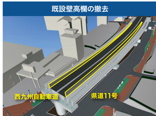
◀既設壁高欄の撤去イメージ
